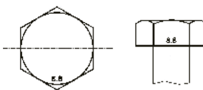
Esempi di marcatura per viti con testa esagonale
