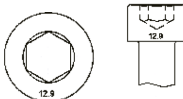
Esempi di marcatura per viti con testa cilindrica e cava esagonale
