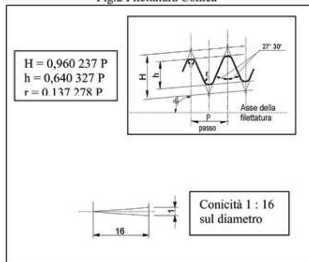
Fig.2 Filettatura Conica
