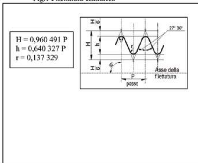
Fig.1 Filettatura cilindrica
